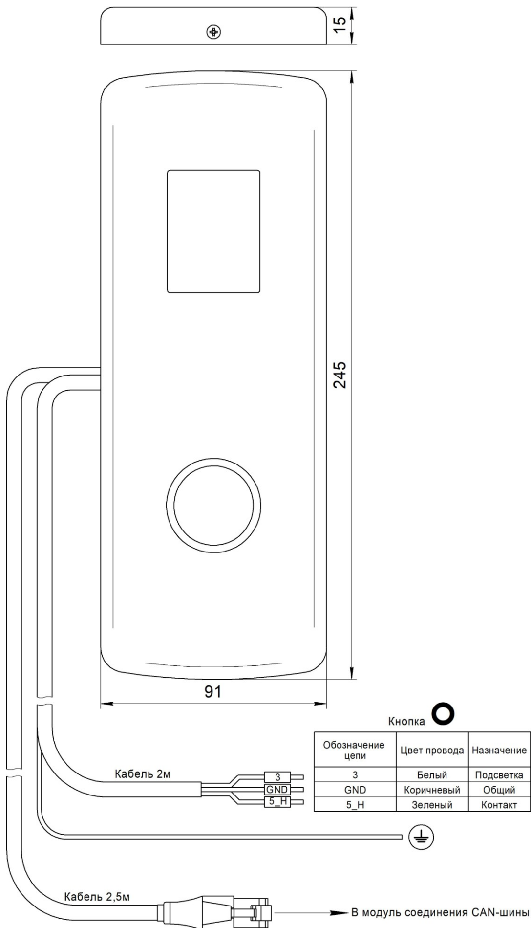
Рис.1 Внешний вид, габаритные и установочные размеры Вызывного поста ЦИРКОН (жгут RJ45) НШЕК.468381.020
